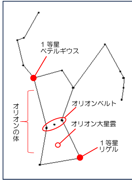
オリオン座
