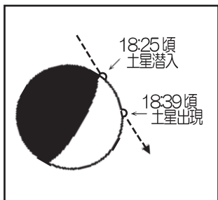
土星食の様子（イメージ）
