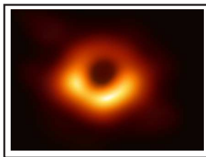
撮影されたブラックホール (Credit:EHTCollaboration)
