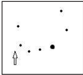
かんむり座 矢印の位置
