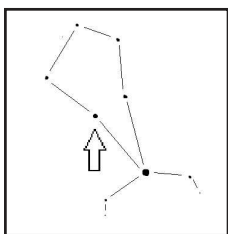
うしかい座 イザールの位置
