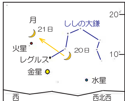
7月21日 20:00 頃の西の空
