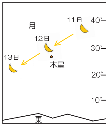
7月中旬 3:00 頃の東の空
