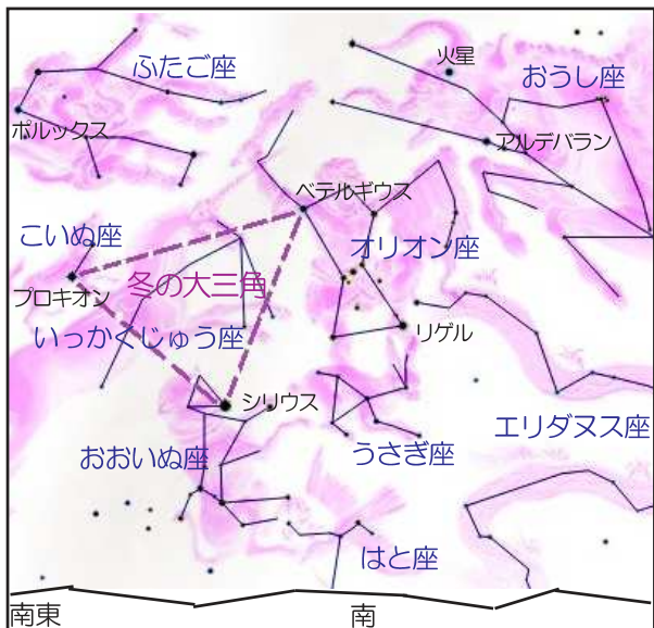
2月中旬20:00頃の冬の星座
