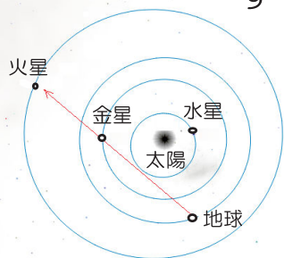
惑星の公転軌道と7月12日の位置
