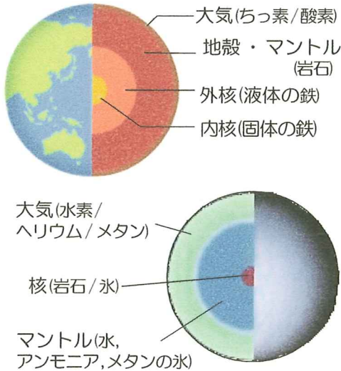
(図)地球(上)と天王星・海王星(下)の構造
