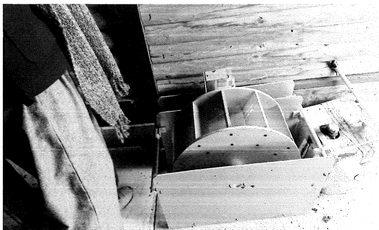
水車の中にある水力発電機
