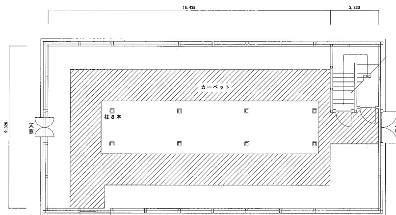
集蔵 平面図 1:100
