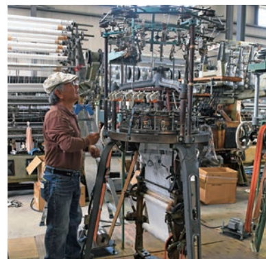
取引先の廃業により譲り受けた「丸編み機」。指導を受けながら、特殊な生産技術を継承している
