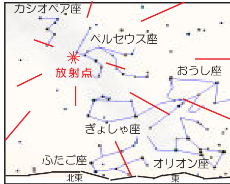
8月13日午前3時頃の空 (イメージ)
