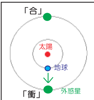
外惑星と地球と太陽の位置関係
